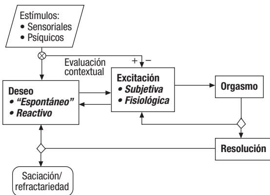
Figura 1. Esquema operativo del ciclo de la respuesta sexual femenina. Frente a los modelos clásicos (como los de Masters y Johnson o Kaplan), que describen sus fases como etapas que se suceden en una secuencia lineal, en la actualidad se prefiere el tipo de interpretación “circular” del estilo de la que se resume en el presente diagrama de flujo 3 . Se pretende resaltar la influencia recíproca entre las distintas fases del ciclo de la respuesta sexual. Así, la reacción de excitación, especialmente en su modalidad subjetiva, que puede ser consecuencia o no (ya que puede precederlo) del estado de deseo, suele reforzar a éste a modo de feedback positivo. También se señala el hecho de que la presentación de una determinada fase no requiere necesariamente la precedente. Por ejemplo, una estimulación sensorial intensa puede producir excitación y hasta orgasmo sin que haya deseo, o incluso cuando exista aversión, lo que puede tener implicaciones psicológicas y legales importantes. Los rombos de decisión tras el orgasmo simbolizan el que éste puede seguirse de la fase de resolución o del retorno a la de excitación que conduzca a una o varias experiencias orgásmicas adicionales antes de entrar en la fase de resolución.
